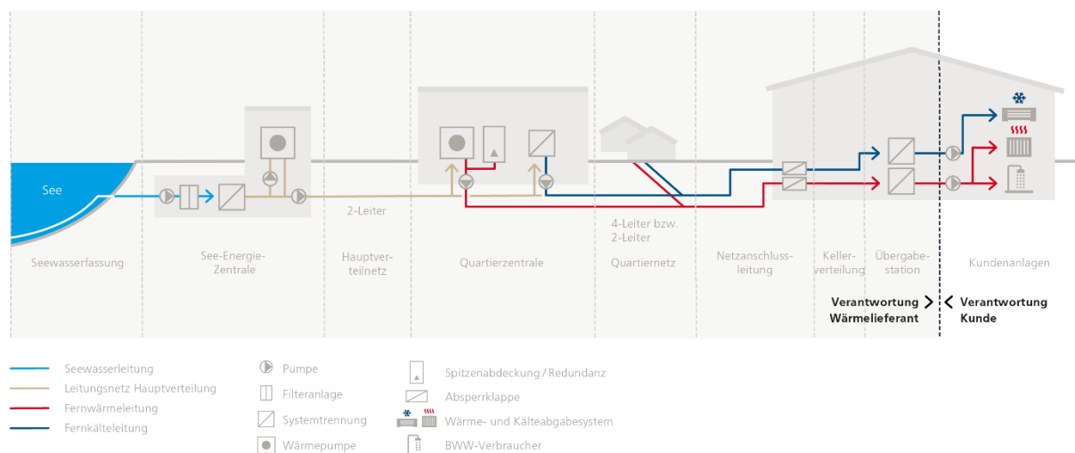
Abbildung 1: Schematische Darstellung des Gesamtsystems mit Quartierzentrale
