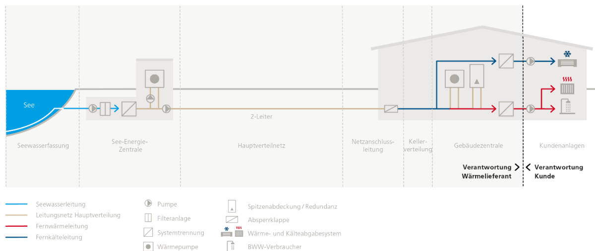
Abbildung 2: Schematische Darstellung des Gesamtsystems mit Gebäudezentrale
